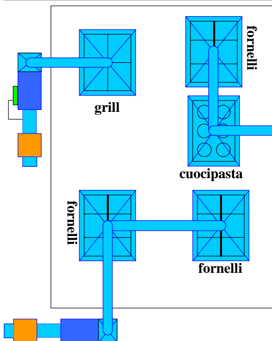
Esempio di intervento su una cucina ospedaliera da 2500 pasti/giorno: quattro unità K da 6000 m 3 /h opportunamente disposte.
